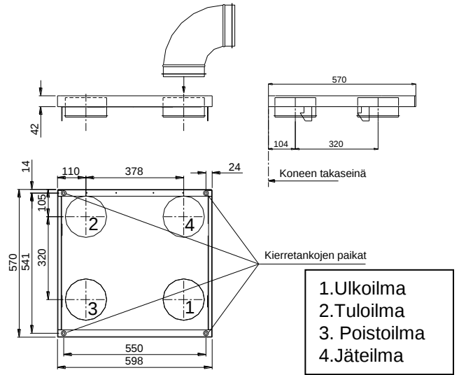
Kuva 5. Kattoasennustelineen mitat (kanavat R-koneeseen)
