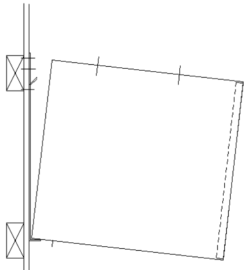
Kuva 4. Seinäasennus
