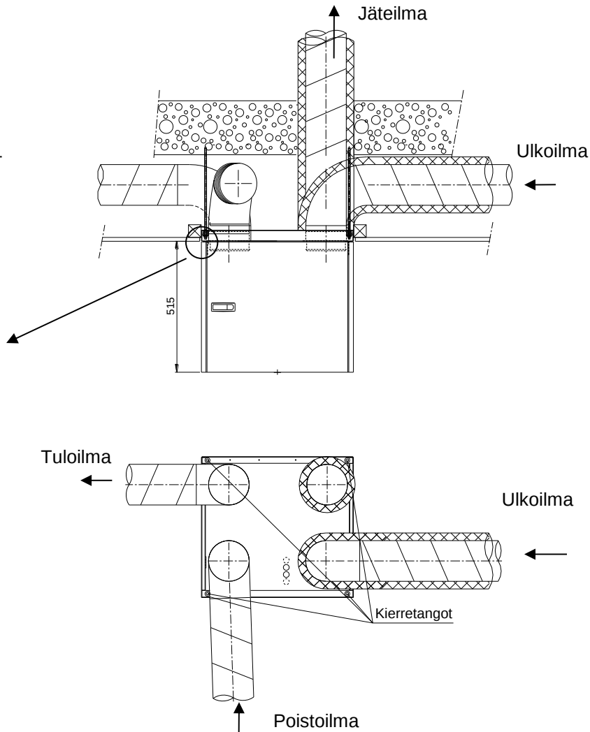
Kuva 5. Kattoasennustelineen mitat (kanavat R-koneeseen)
