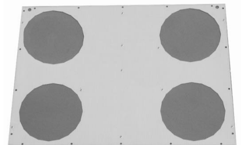
Kuva 2. Höyrysulun läpivientilevy
